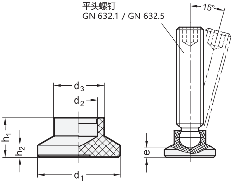
装配示例
